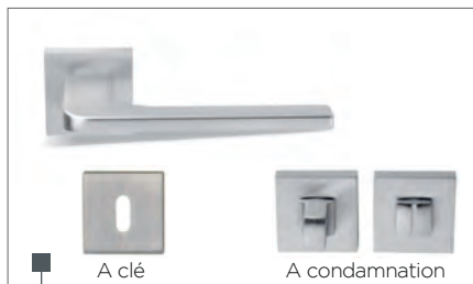
ARYA - Kit poignée rosace carrée Encombrements : 140 x 55 mm. 2 coloris : Chrome satiné et Noir.
